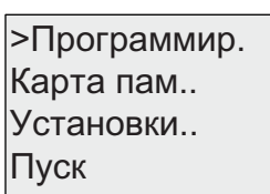
Главное меню модуля LOGO!
