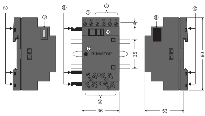
Модуль расширения LOGO! (например, DM8 12/24 R)
