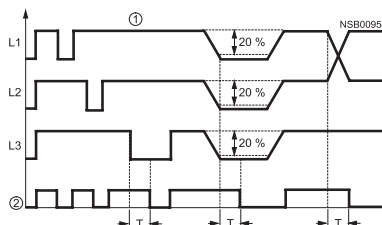
① Измеряемое напряжение U_n ② Выходное реле
