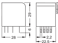
Промышленное реле LZX:PT570
