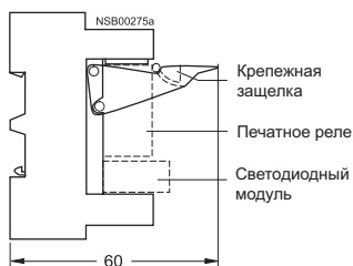
Комплетное устройство LZX:RT3/RT4
