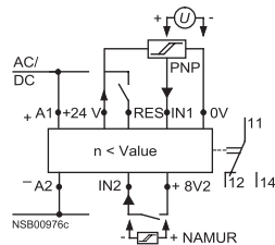
Реле контроля снижения частоты вращения 3UG30 51
