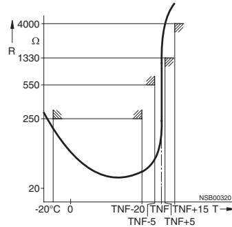
Графики температурных датчиков типа А описаны в нормах МЭК 600.4-11-2 (DIN VDE 0660 часть 303), DIN 44081 и DIN 44082.
