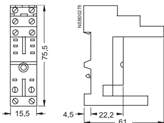
Втычной цоколь LZX:RT78626 С безопасной развязкой для печатного реле
