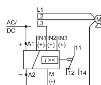
Реле контроля тока, однофазное 3UG35 21, 3UG35 22
