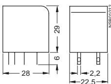
Промышленное реле LZX:PT270
