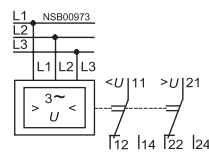
Реле контроля напряжения, трехфазное 3UG30 41
