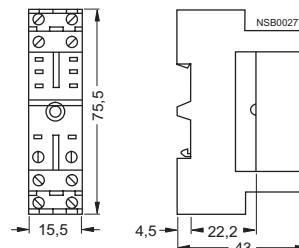
Втычной цоколь LZX:RT78625 Для печатного реле
