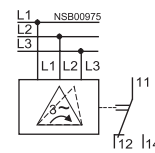
Реле контроля асимметрии, трехфазное 3UG30 12
