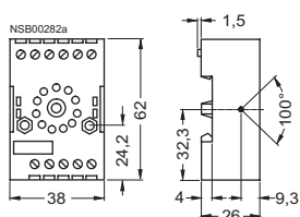
Втычной цоколь LZX:MT78750 Для промышленного реле
