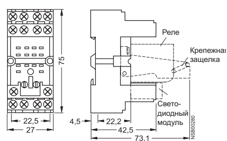
Втычной цоколь LZX:PT78704 Для промышленного реле
