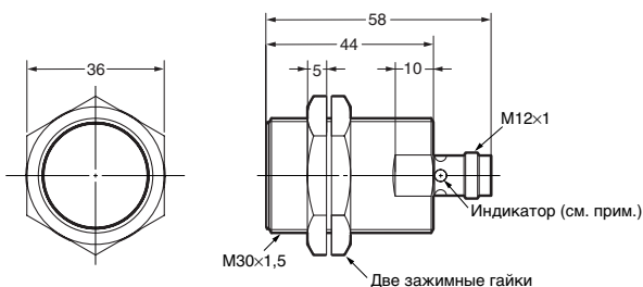
E2A-M30KS15-M1-□□/E2A-S30KS15-M1-□
